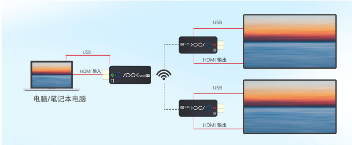
ASK nano 4K（1 发 2 收）系统连接简图
