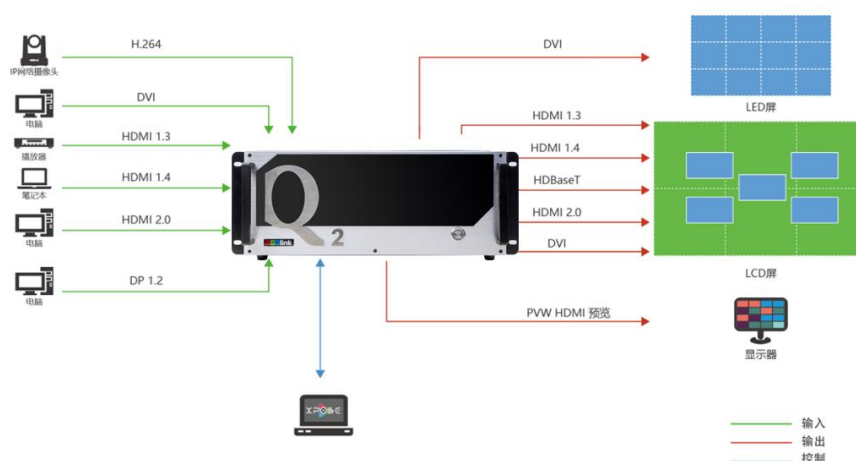
Q2 Gen2 4U 的系统连接简图
