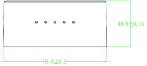
右视图
