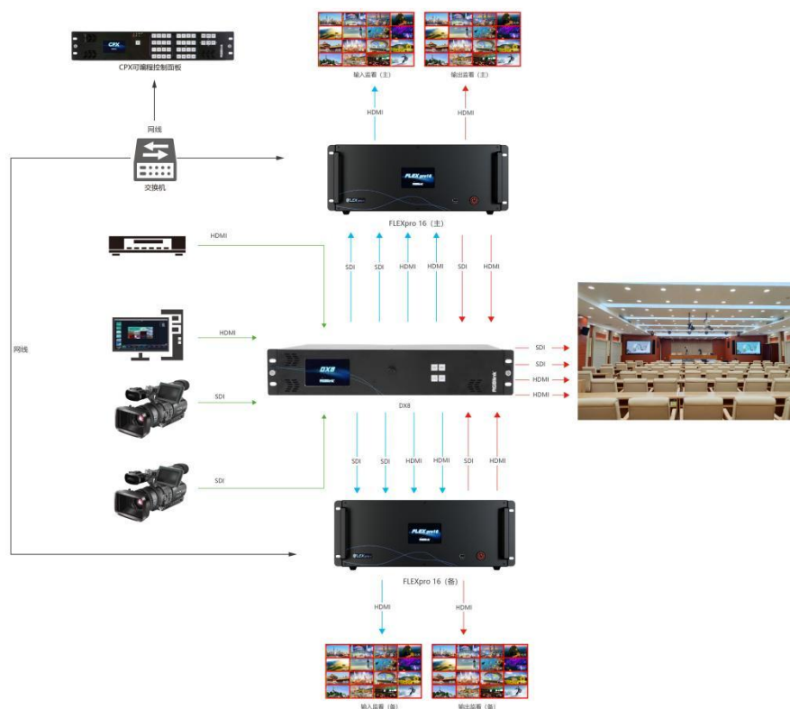
FLEXpro16 的系统连接图
