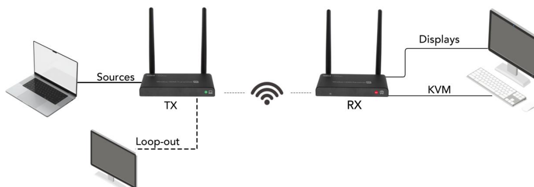
图为 ASK plus p2p 的系统连接简图
