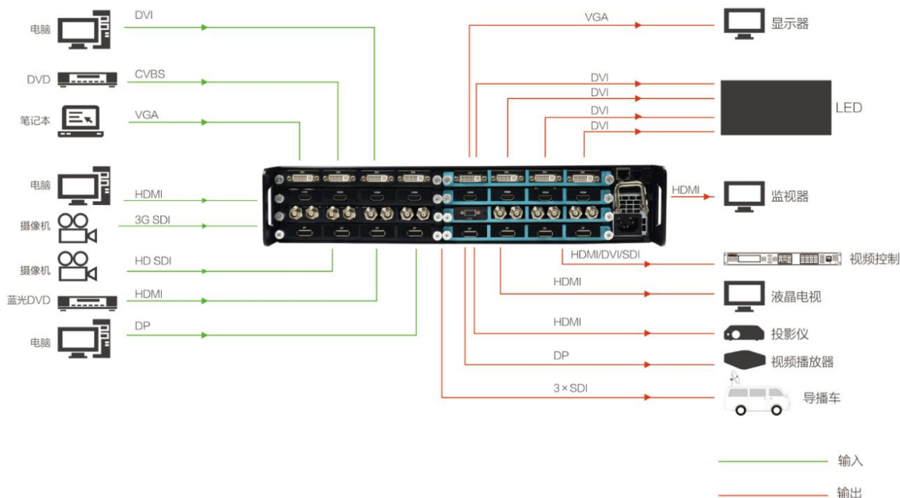
FLEX 16 系统连接简图
