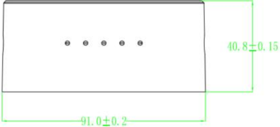
右视图
