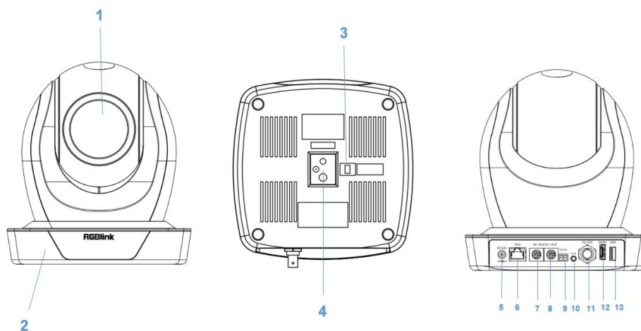
图 2.1 PTZ 摄像头外部接口
