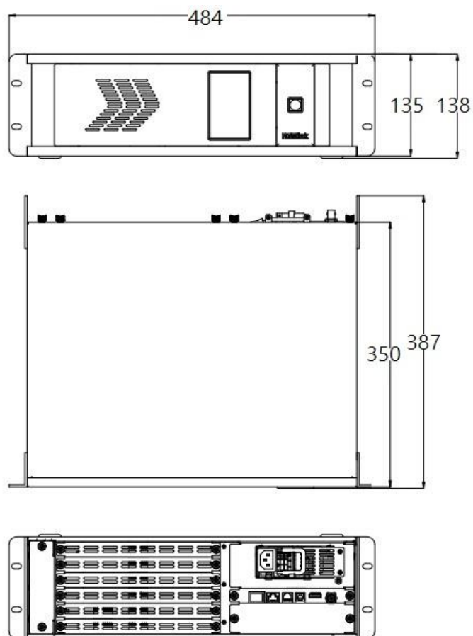
图为X3，尺寸单位:mm
